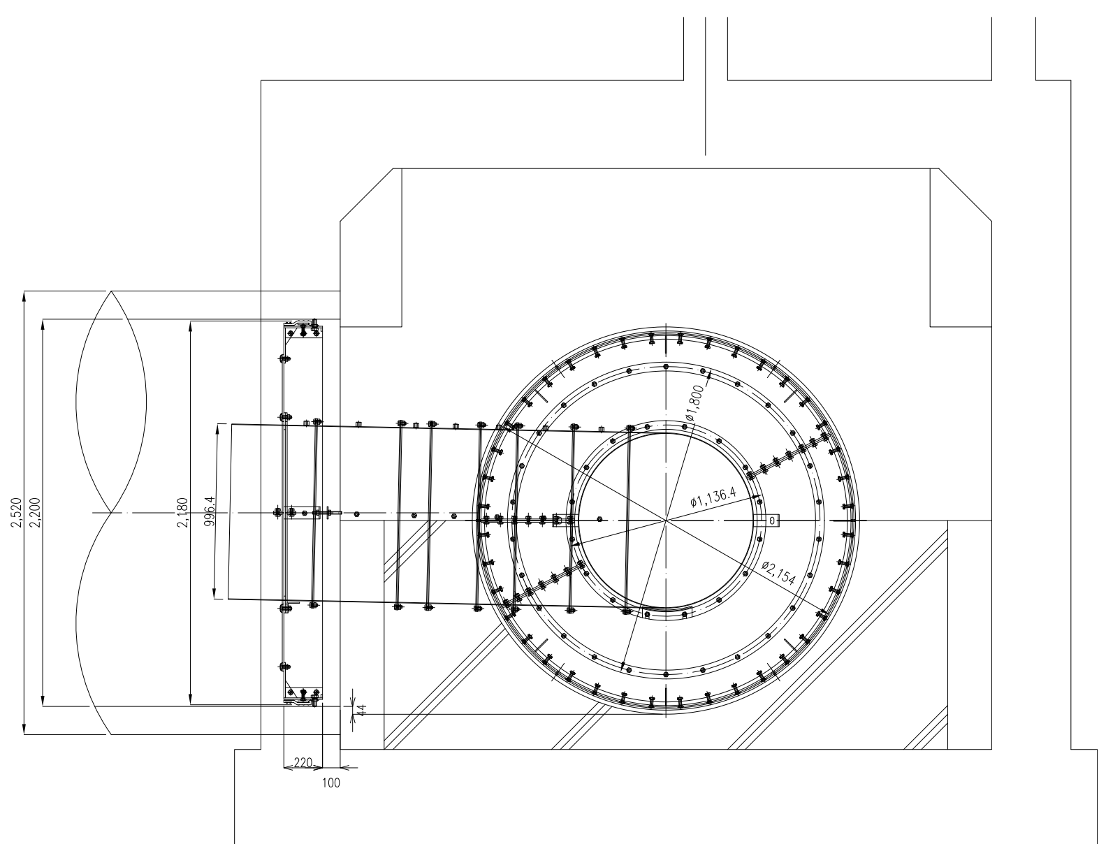
図名 N県 プラグ設置図 スーパープラグφ2200上下流 バイパス管φ1000 79° 43' 落差44
